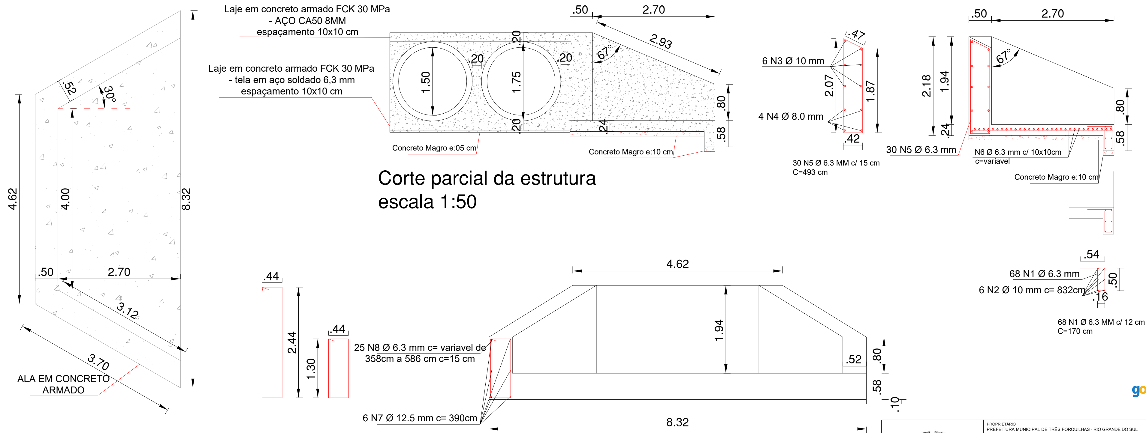
Detalhamento Encontro escala 1:50
