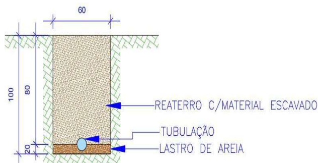
DETALHAMENTO VALA REDES PRINCIPAL
