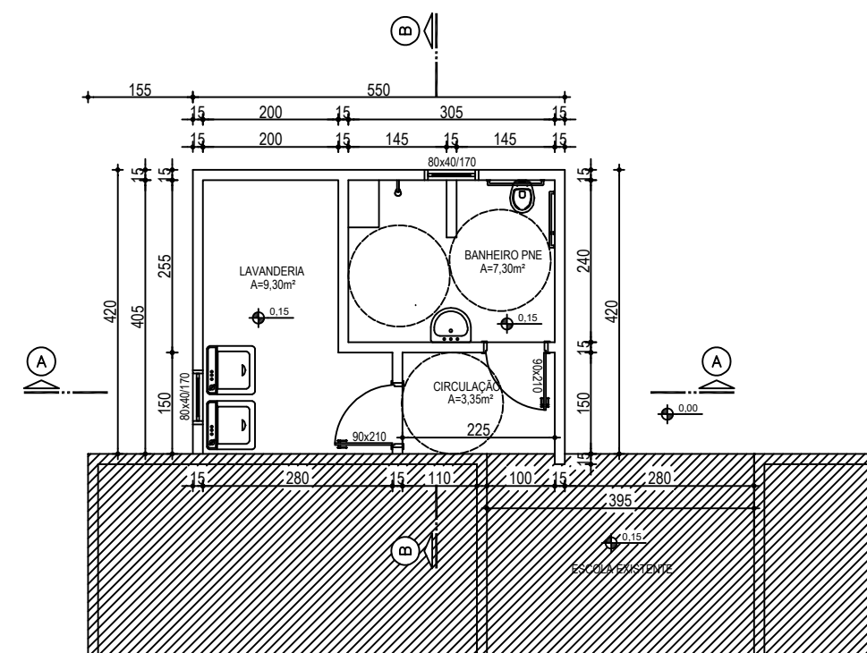
PLANTA BAIXA Area: ____ 23,10m² Escala: ____ 1/100
