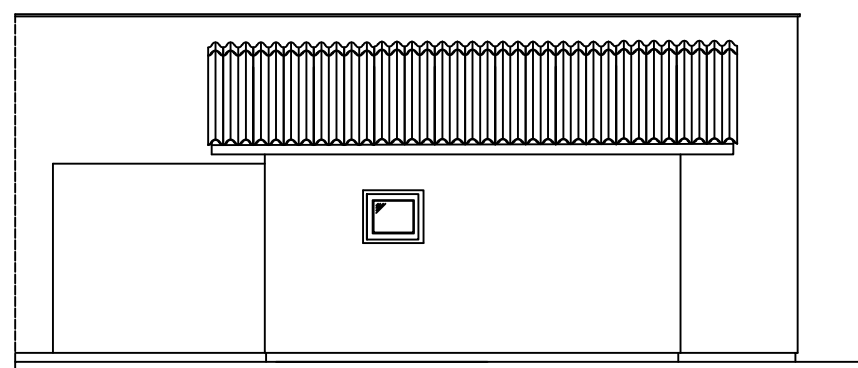
Fachada Oeste Escala: ____ 1/100
