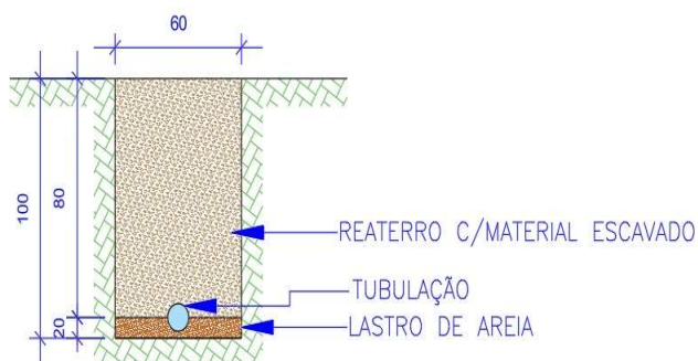
DETALHAMENTO VALA REDES PRINCIPAL
